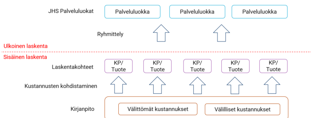
Kuva 3. Kustannuslaskenta ideaalitalanteessa.
